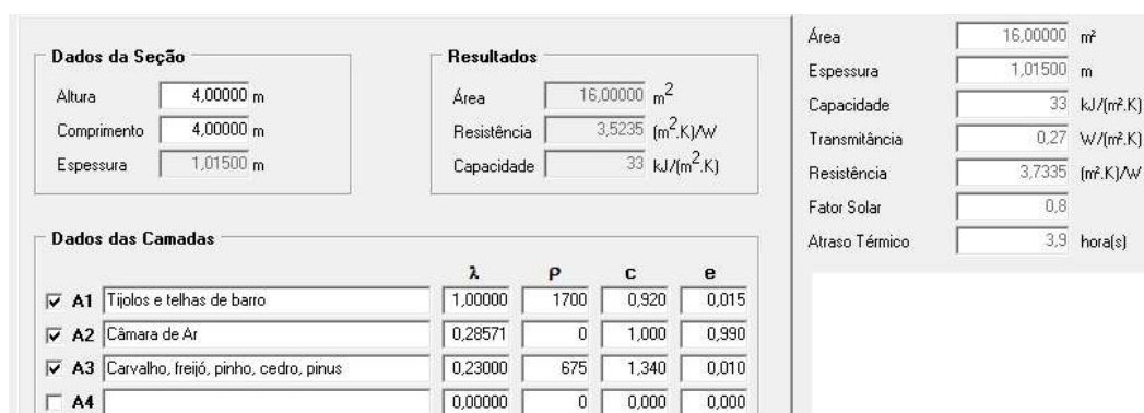
FIGURA 07 - CONSIDERAÇÕES DAS CAMADAS DA COBERTURA
