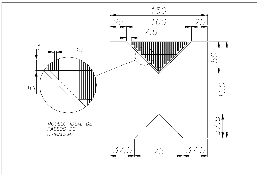
FIGURA 2: PERFIL DO PRODUTO CONFORME NOVO MÉTODO DE DESBASTE FONTE: OS AUTORES (2013)
