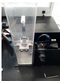
FIGURA 4: MONTAGEM FINAL DO DISPOSITIVO MECÂNICO DE TESTE JATO D'ÁGUA FONTE: O AUTOR (2018)
