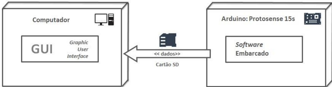
FIGURA 1 - DIAGRAMA DE IMPLANTAÇÃO DO PROJETO FONTE: CRIADO PELO AUTOR
