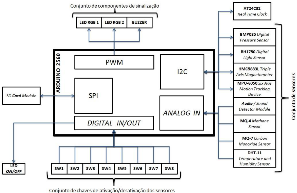
FIGURA 2 - DIAGRAMA DE BLOCOS FUNCIONAIS DO PROTÓTIPO FONTE: CRIADO PELO AUTOR
