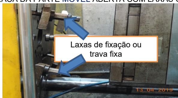
FIGURA 4 - PLACA DA PARTE MÓVEL ABERTA COM LAXAS OU TRAVA FIXA
